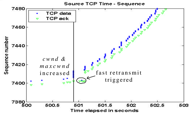
TCP SACK + QA: GPRS->WLAN src TCP
