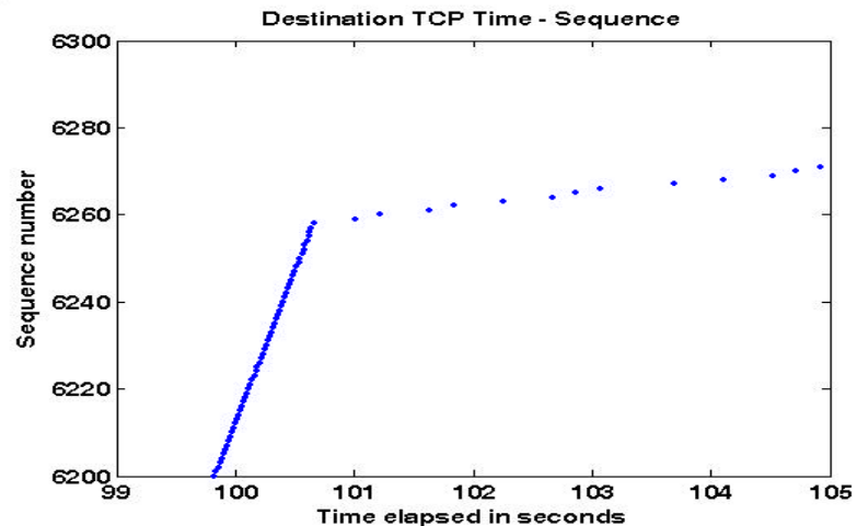
TCP SACK + QA: WLAN->GPRS dst TCP
