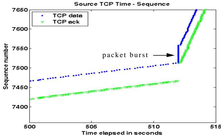
TCP SACK: GPRS->WLAN src TCP
