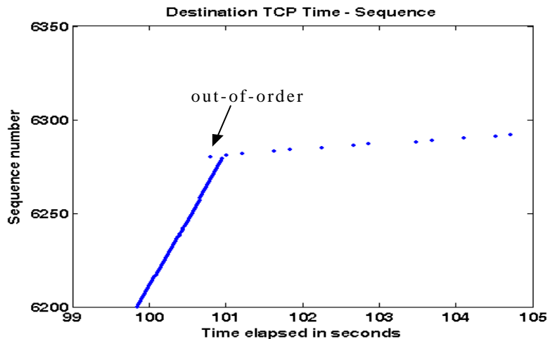
TCP SACK: WLAN->GPRS dst TCP
