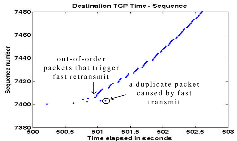
TCP SACK + QA: GPRS->WLAN dst TCP
