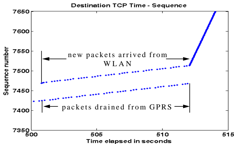
TCP SACK: GPRS->WLAN dst TCP
