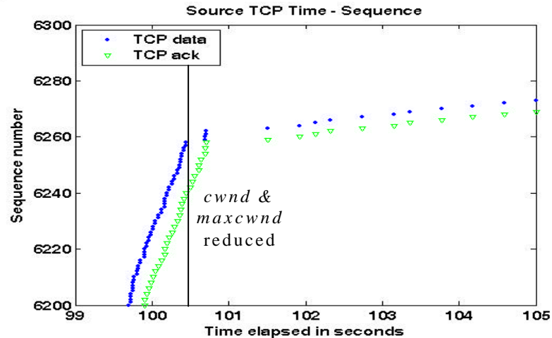
TCP SACK + QA: WLAN->GPRS src TCP
