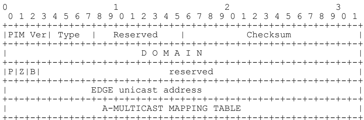
Figure 40 PER introduction message
